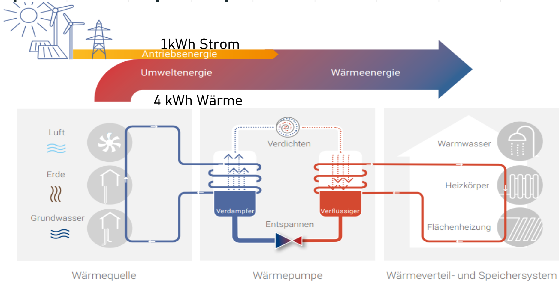
Abb. 2: Funktionsprinzip Wärmepumpen
